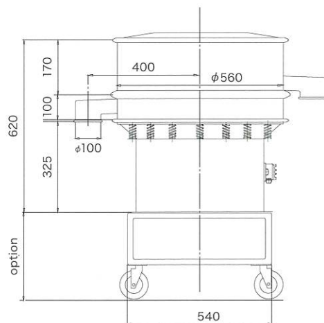
LS-600-1S 主寸法
